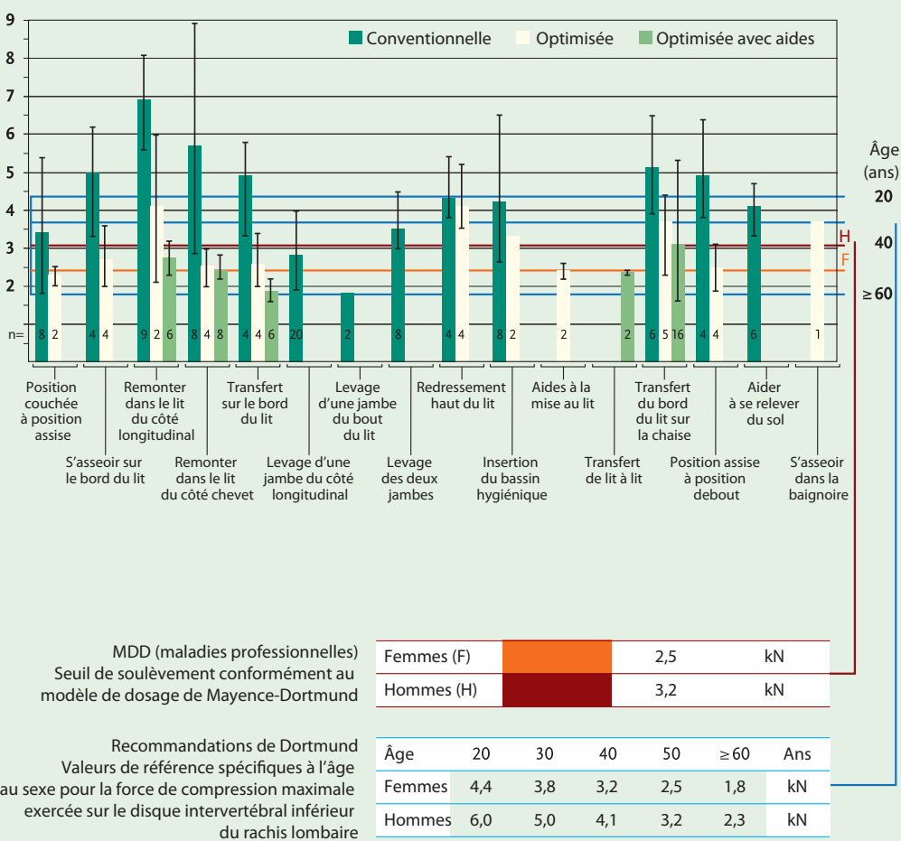
Force de compression exercée sur le disque intervertébral inférieur du rachis lombaire (L5-S1) en kilonewton (kN)
